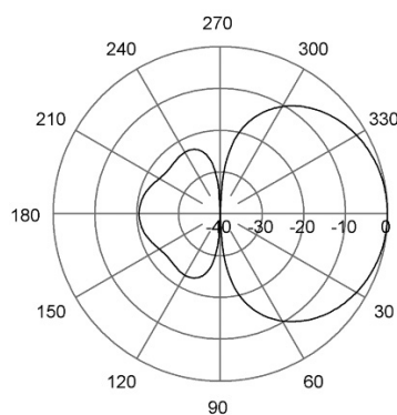
E-Plane | 165 MHz
