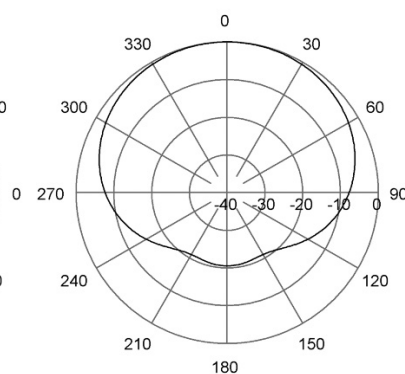
H-Plane | 165 MHz
