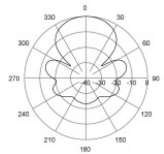
H-Plane | 155 MHz
