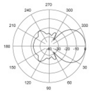
E-Plane | 155 MHz
