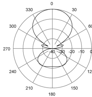
E-Plane | 148 MHz
