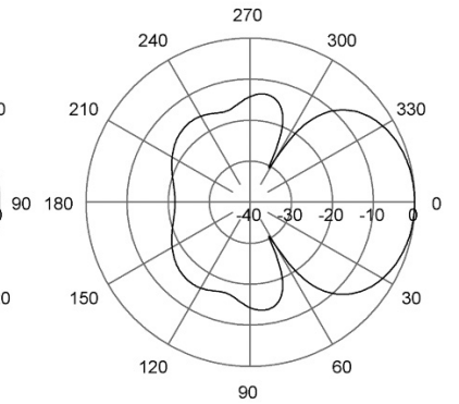
H-Plane | 148 MHz
