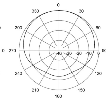
H-Plane | 153 MHz
