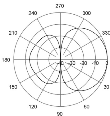
E-Plane | 153 MHz
