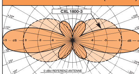
TYP. STRAHLUNGSDIAGRAMM (VERTIKAL)
