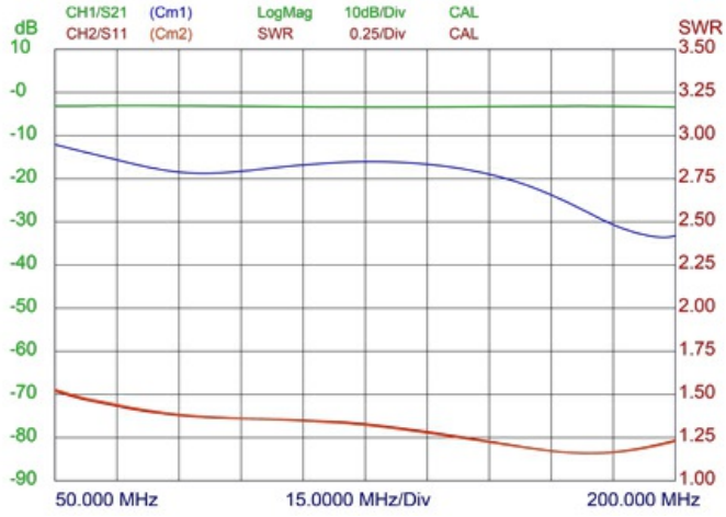
Typischer kurvenverlauf für 3 dB
