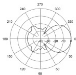
E-Plane | 445 MHz
