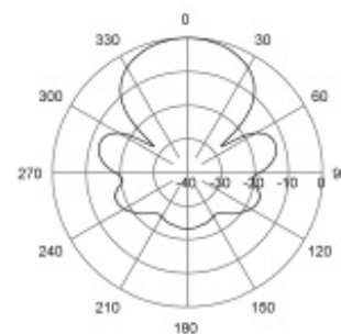
H-Plane | 445 MHz
